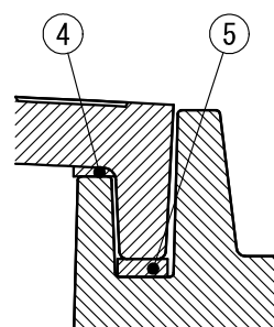
Q部拡大図 (1/2)
