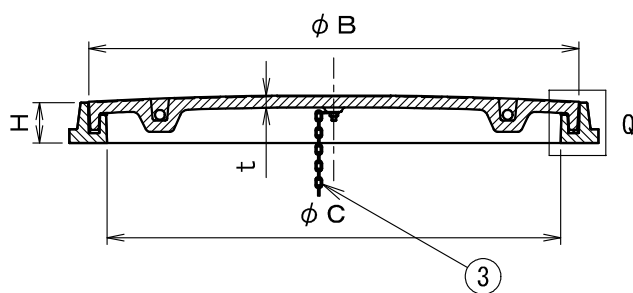
A-A 断面図
